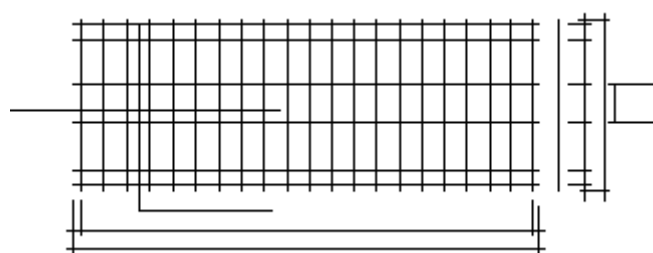
Z5-1. Siatka zbrojenia podporowego P-1 kliknij, aby powiększyć
