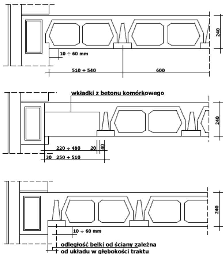
Z6-2. Sposób układania pustaków przy ścianach równoległych do belek
