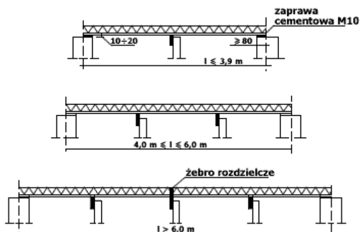
Z6-1. Sposób podpierania belek
