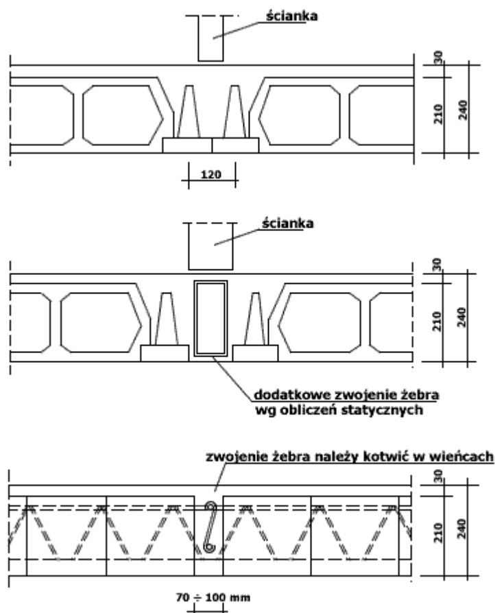
Z6-3. Przykład rozwiązania wieńców stropowych
